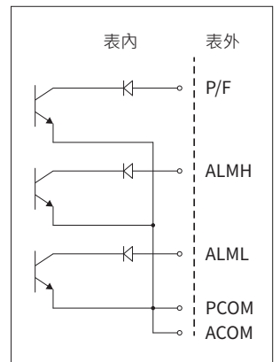
頻率輸出內部電路
